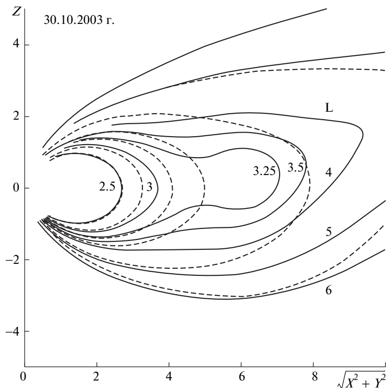
Рис. 4. Расчет конфигурации магнитных силовых линий. По оси ординат – Rz – расстояние от плоскости магнитного экватора в земных радиусах в геомагнитных координатах, по оси абсцисс – расстояние от центра Земли в плоскости X-Y . L от 2.5 до 6 (см. табл. 2). Сплошные линии относятся к пролету спутника на ночной стороне (MLT = 20.10), пунктирные – к примыкающему пролету на дневной стороне (MLT = 08.15), линия L = 3.25 пропущена.
