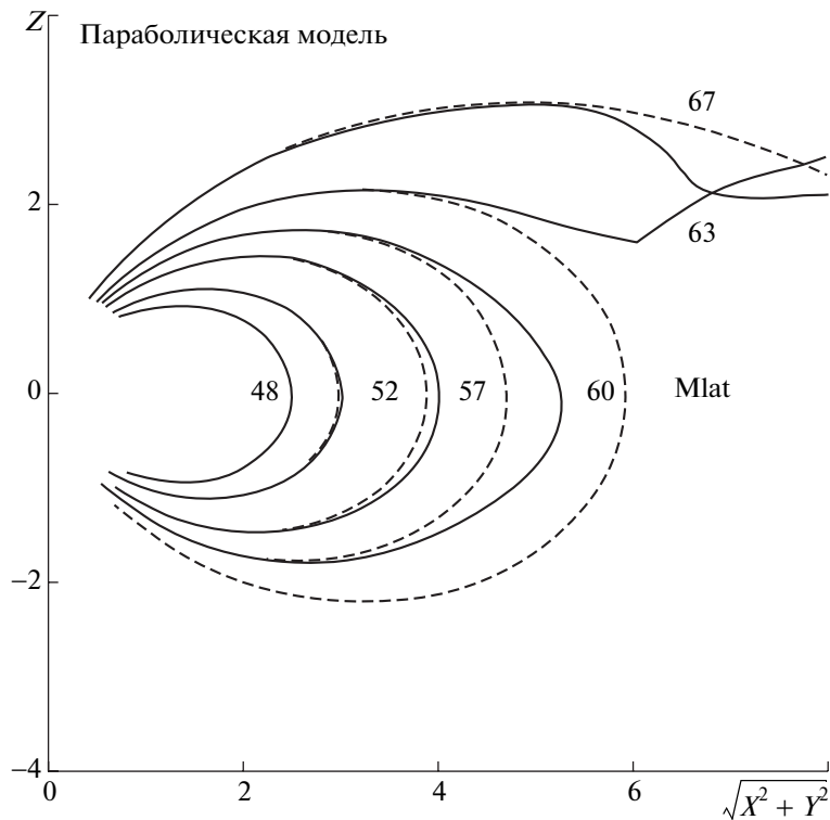
Рис. 9. Конфигурация силовых линий магнитного поля 29.10.2003 г., рассчитанная по параболической модели, ночной и дневной (пунктир) сектора.
