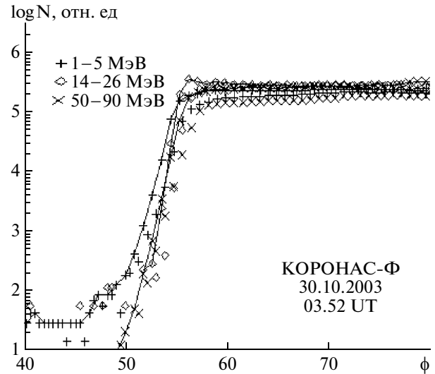
Рис. 2. Широтный профиль протонов СКЛ 30.10.2003 г. По оси абсцисс — геомагнитная широта, по оси ординат — интенсивность протонов, выровненная по измерениям в полярной шапке. Сплошные линии со знаками — ночной пролет, отдельные значки — дневной.
